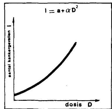
Kwadratisch model
