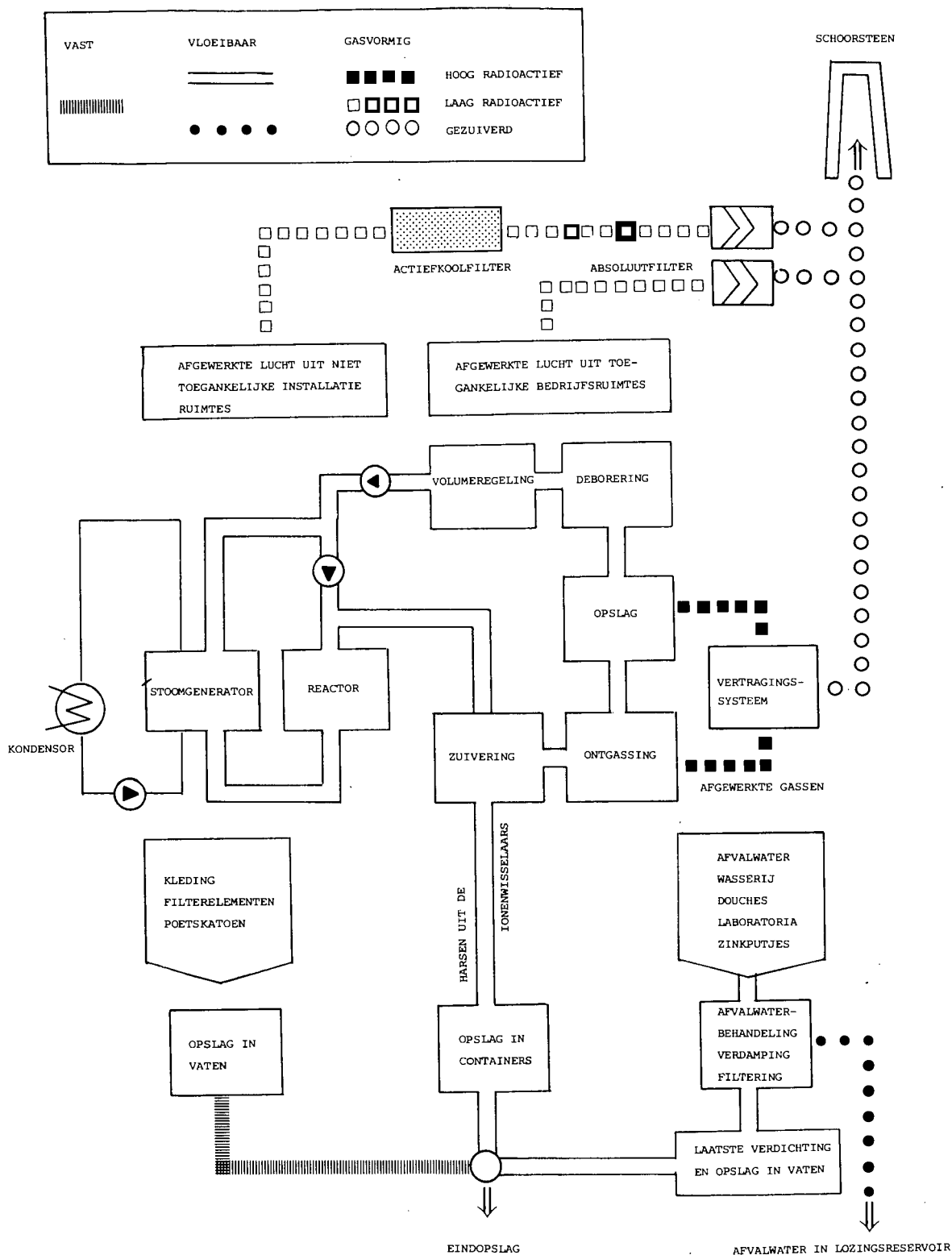
Figuur 4.1 Stroomschema van de radioactieve stoffen in de kerncentrale te Lingener. (uitgezonderd reactorkern) (ref. 7.)
