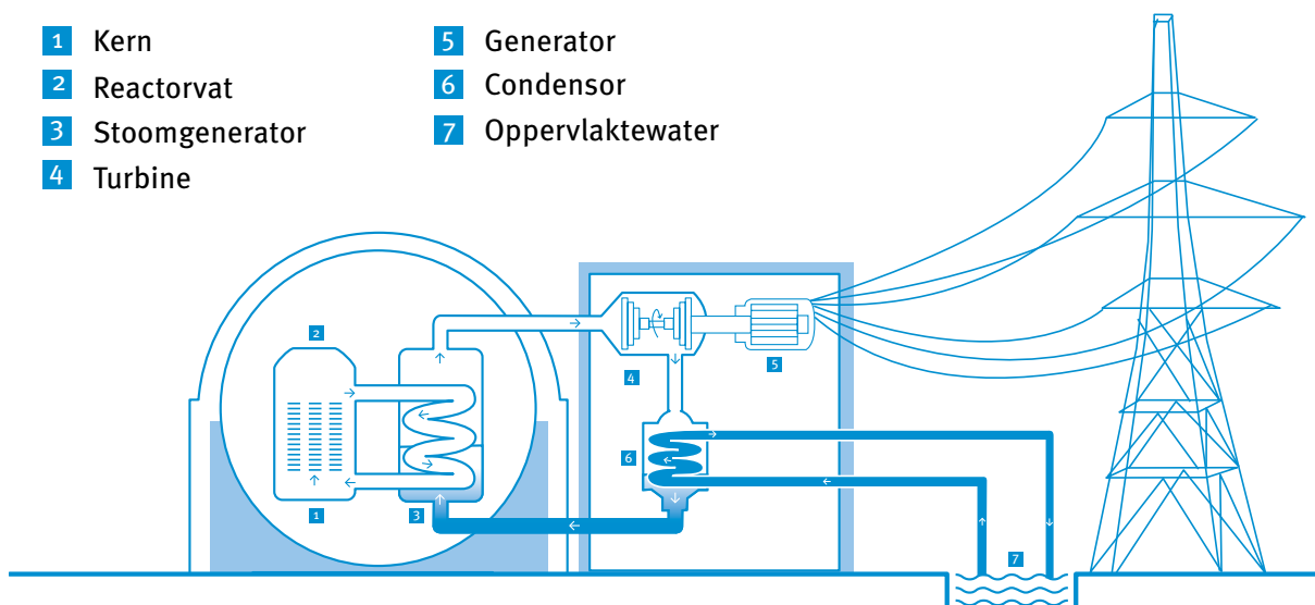
Figuur 5: Principeschema van een lichtwater drukreactor
