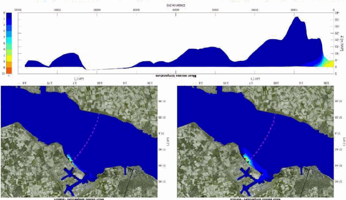
Figuur B.4 Gesimuleerde gemiddelde temperatuurstijgingsvoetdruk als gevolg van de bestaande warmteinzettingen en de nieuwe Borssele 2-lozing (Scenario03).
