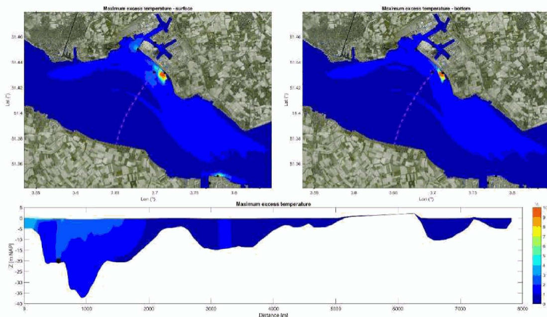
Figuur 4.32 Gesimuleerde maximum temperatuurstijgingsvoetafdruk als gevolg van de bestaande warmtelozingen én de nieuwe Borssele 2-lozing (Lozingsoptie 3 en Configuratie 7).
