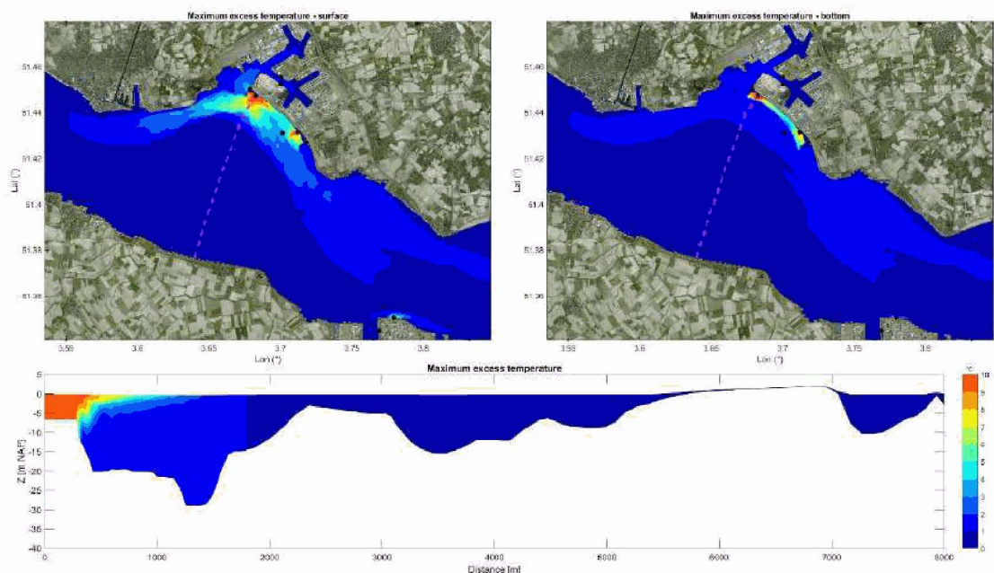
Figuur 4.21 Gesimuleerde maximum temperatuurstijgingsvoetafdruk als gevolg van de bestaande warmtelozingen én de nieuwe Borssele 2 lozing (Configuratie 6).
