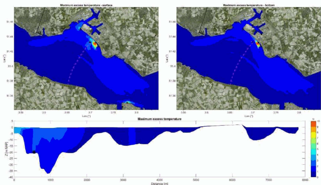
Figuur 4.31 Gesimuleerde maximum temperatuurstijgingsvoetafdruk als gevolg van de bestaande warmtelozingen én de nieuwe Borssele 2-lozing (Lozingsoptie 2 en Configuratie 7).
