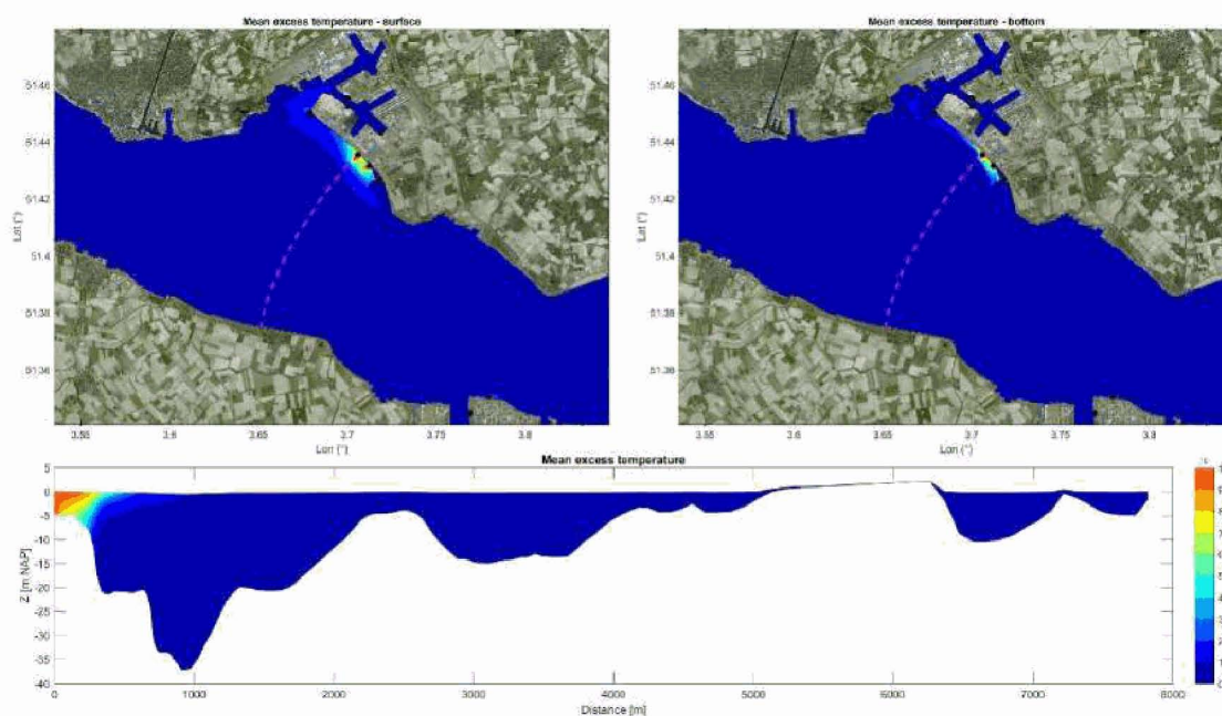
Figuur B.2 Gesimuleerde gemiddelde temperatuurstijgingsvoetafdruk als gevolg van de bestaande warmtelozingen én de nieuwe Borssele 2-lozening (Scenario01).
