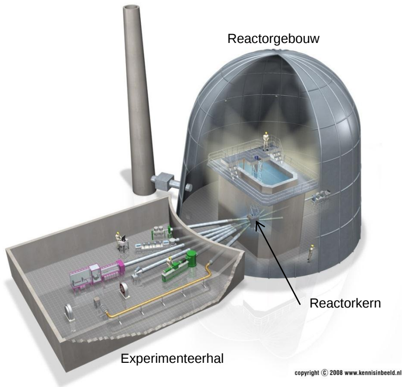
Figuur 1 Doorsnede van het reactorgebouw en de experimenteerhal
