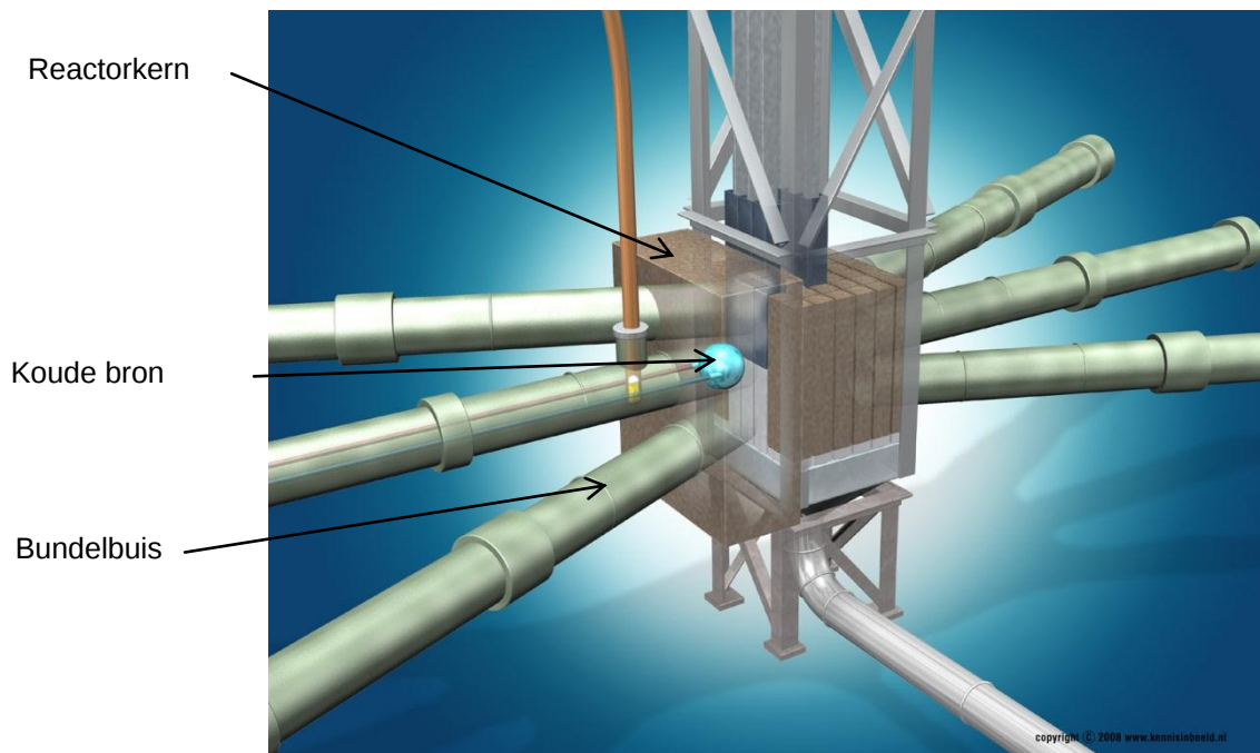
Figuur 2 Reactorkern met bundelbuizen en koude bron
