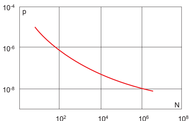
Obr. č. 1: Střední maximální dovolená pravděpodobnost závažných havárií p v závislosti na celkovém počtu reaktorů N
