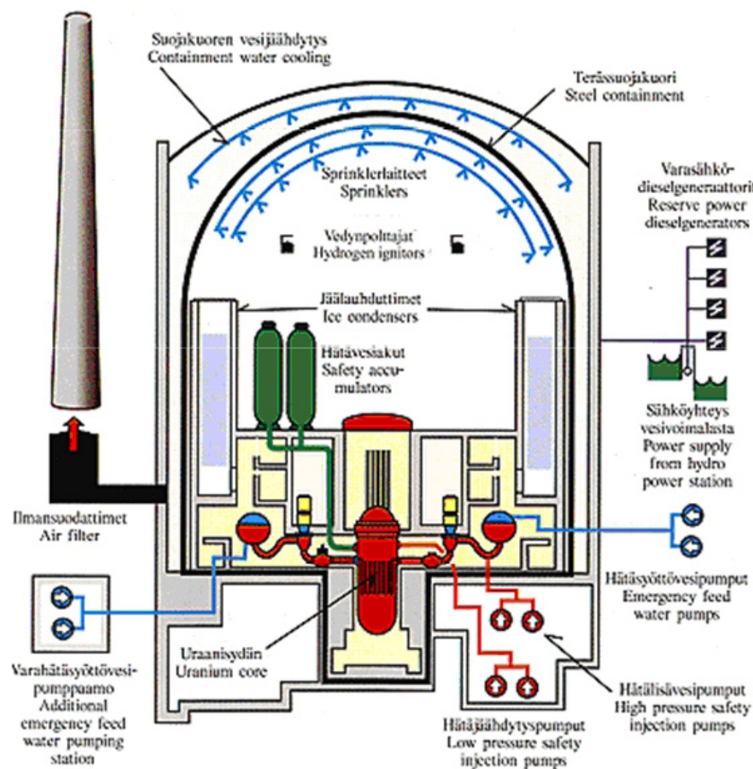
Obr. č. 4: Bezpečnostní systémy JE Loviisa
