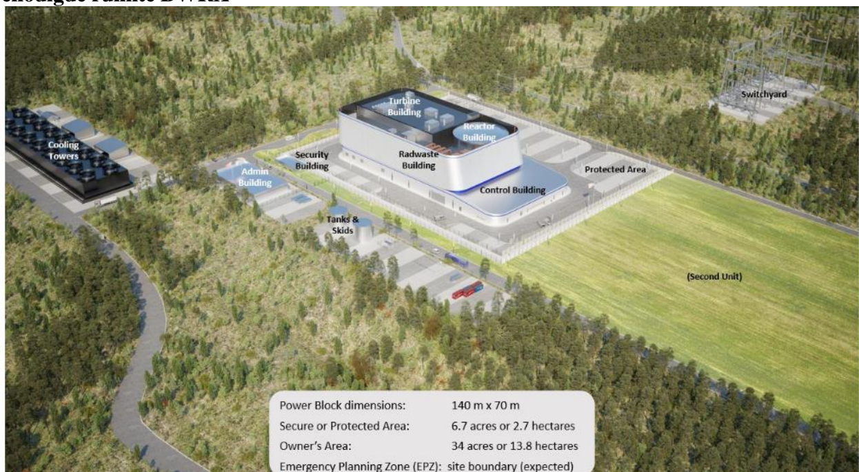
Figuur 4 Benodigde ruimte BWRX
