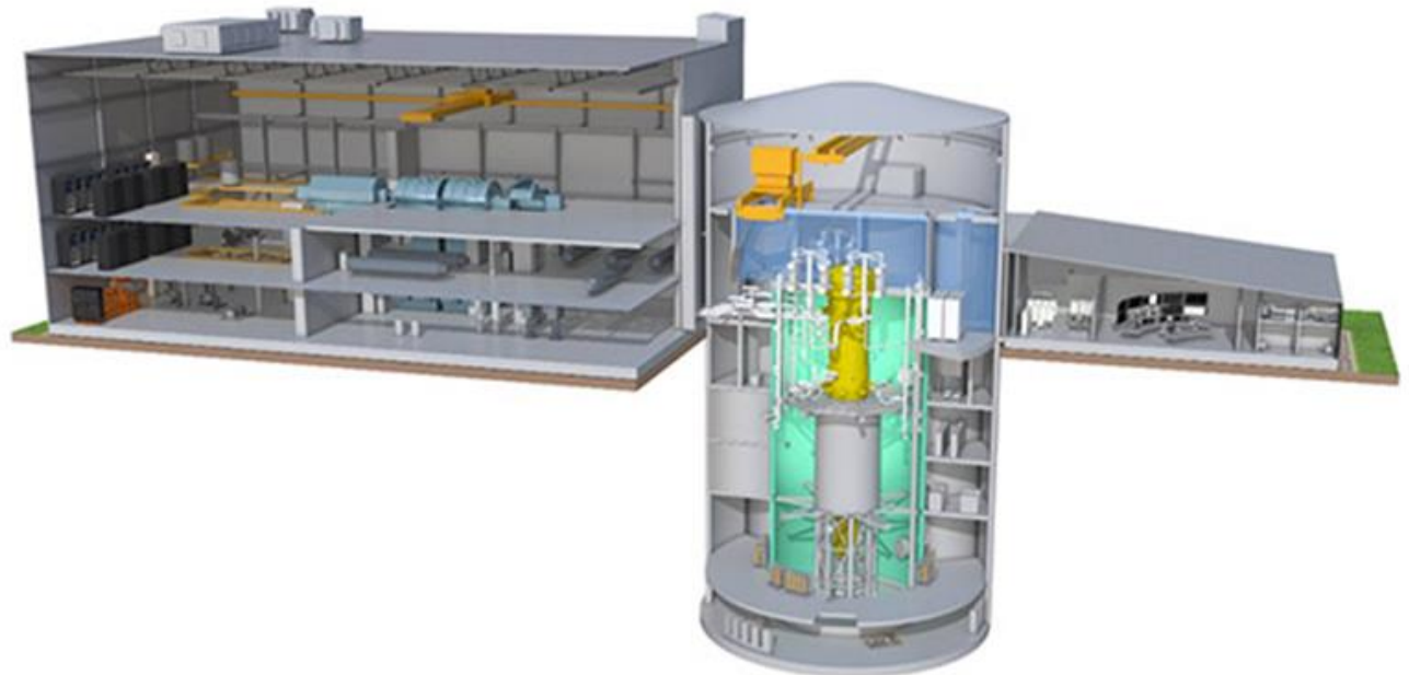
Figuur 2 Doorsnede BWRX
