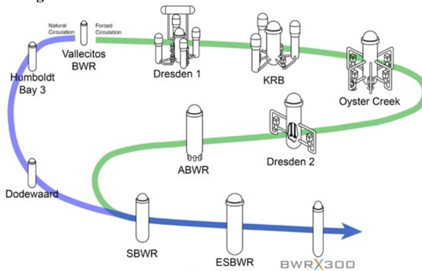
Figuur 4 Ontwikkeling kokend-water-kerncentrales vanaf 1960
