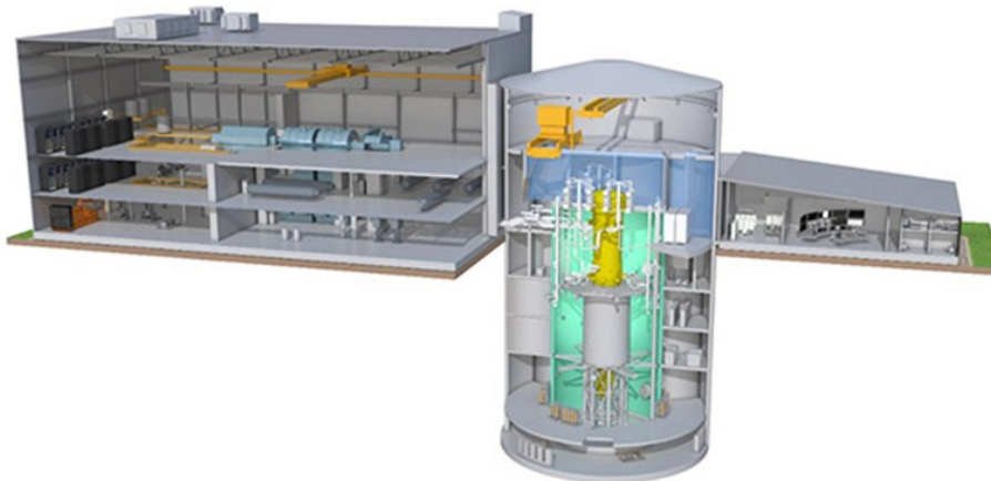
Figuur 3 Doorsnede BWRX
